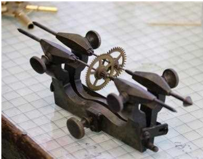
Engrenagepasser klein model met twee ingeklemde uurwerkkraden
