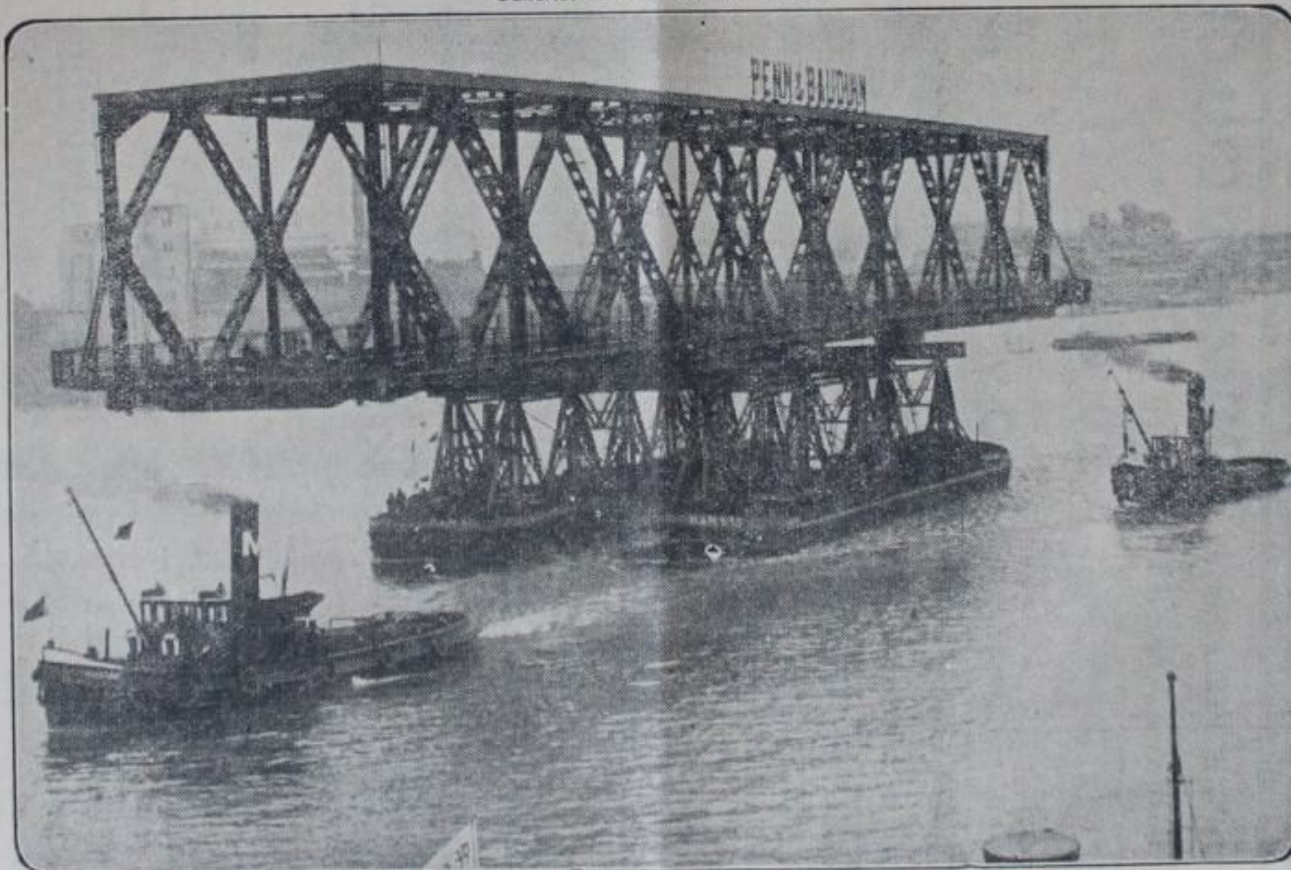
De tweede spanning voor de brug over het Hollandsch Diep aan den Moerdijk is Woensdag van Dordrecht naar de plaats van bestemming gebracht. — Het transport onderweg
