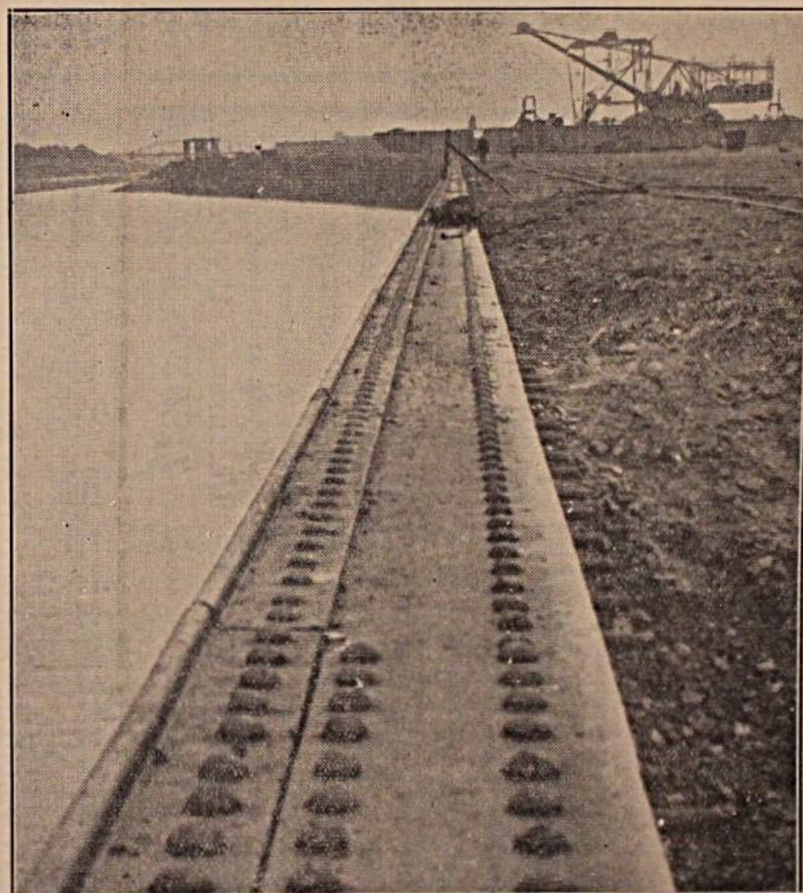
De haven der staatsmijnen te Stein is thans geheel voltooid. — Op den achtergrond de werkzaamheden voor den bouw van den tip voor het overladen der kolen
